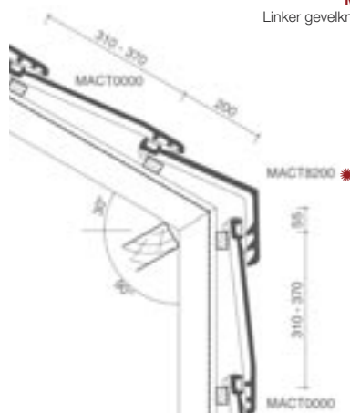
Lengtedoorsnede dak met gevel ter hoogte van knikpan
