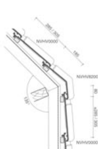
Lengtedoorsnede dak met gevel ter hoogte van knikpan
