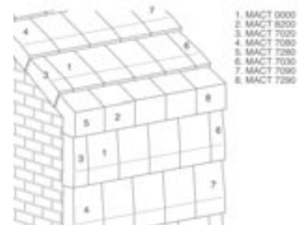
3D tekening met knikpan
